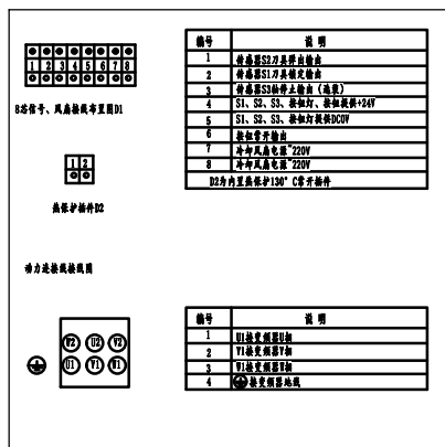
JGL-9.0K 接线图
