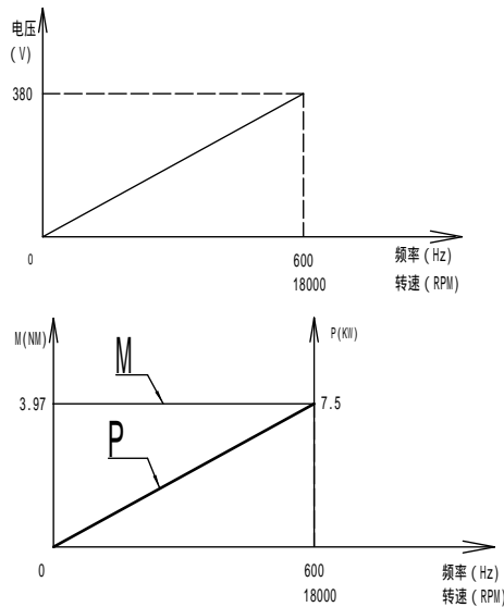
JGL-7.5K电主轴曲线图
