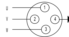
接线图
