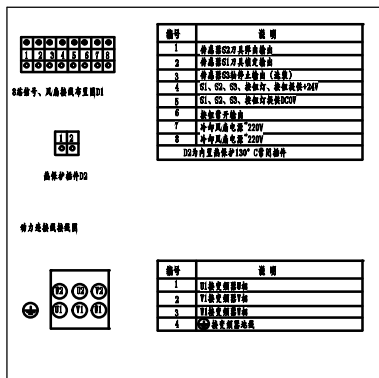
接线图
