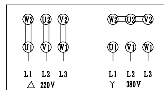
接线图
